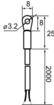
Габаритный размер датчика
